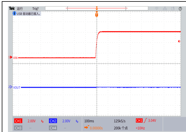
短路保护
