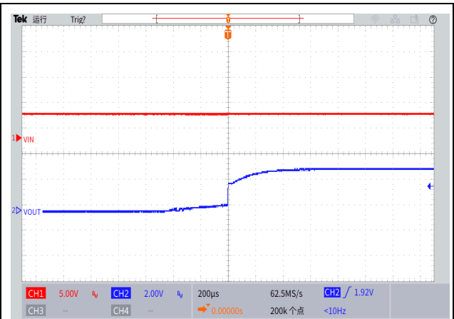
短路恢复
