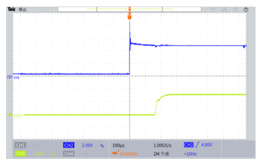
图 3 快上电 (VIN=5V IOUT=0mA)
