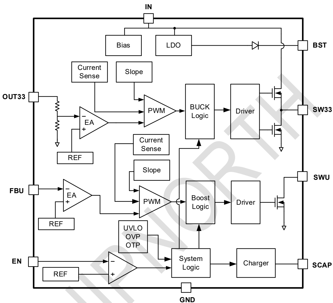
图 4 功能框图
