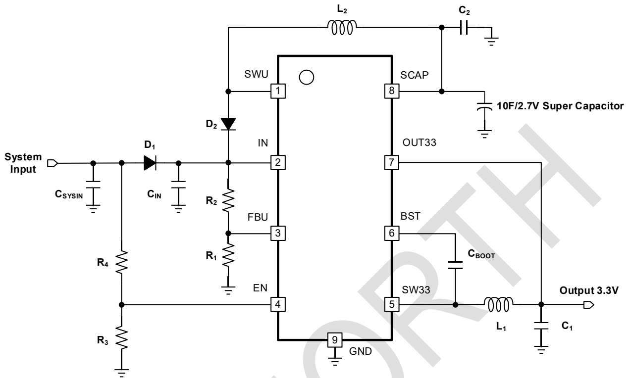
图 3 典型应用
