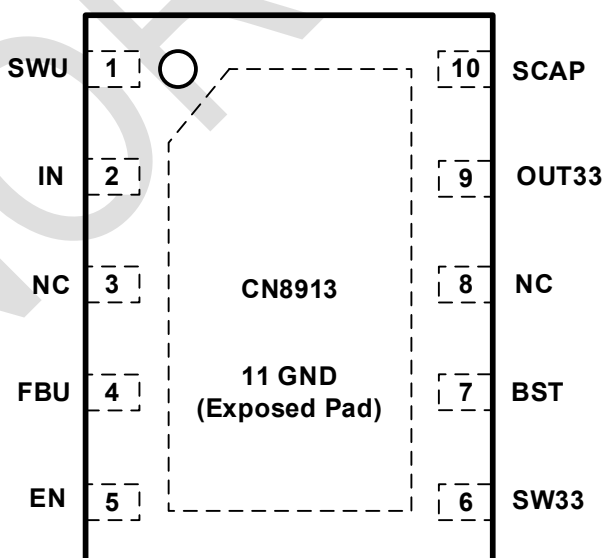
图 2 DFN3X3-10L
