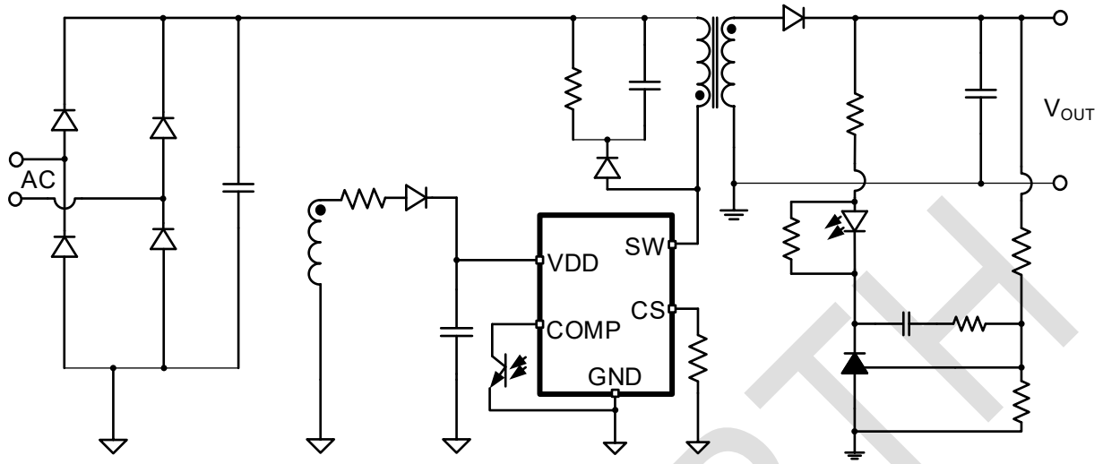
CN12039A、CN12039B 典型应用图
