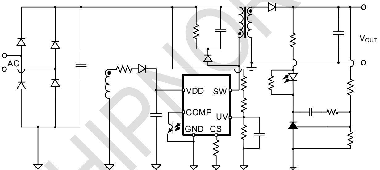
CN12039C、CN12039D 典型应用图
