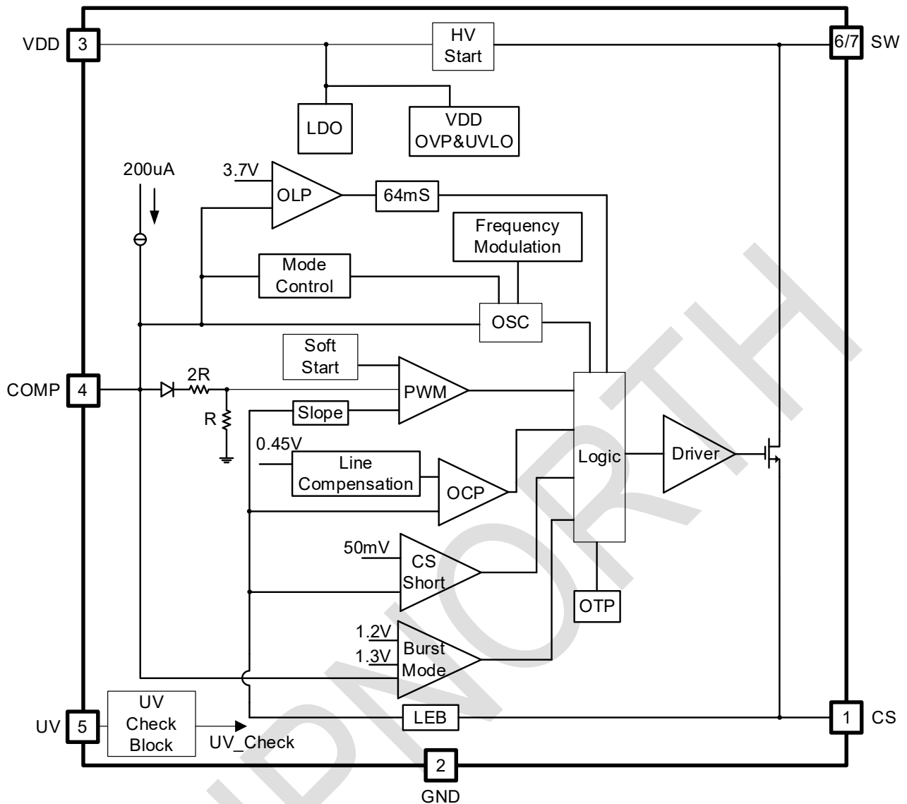
CN12039C、CN12039D 功能框图
