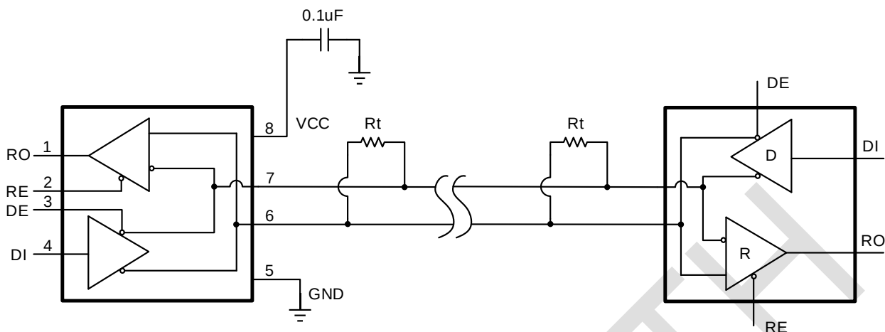
RS485 典型半双工工作电路
