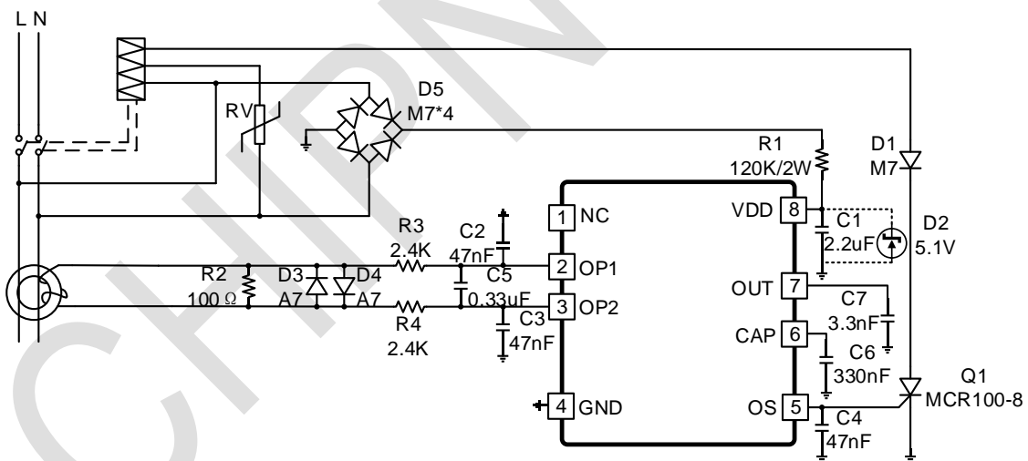
图 6.2 CN54124B/C/D 典型应用图
