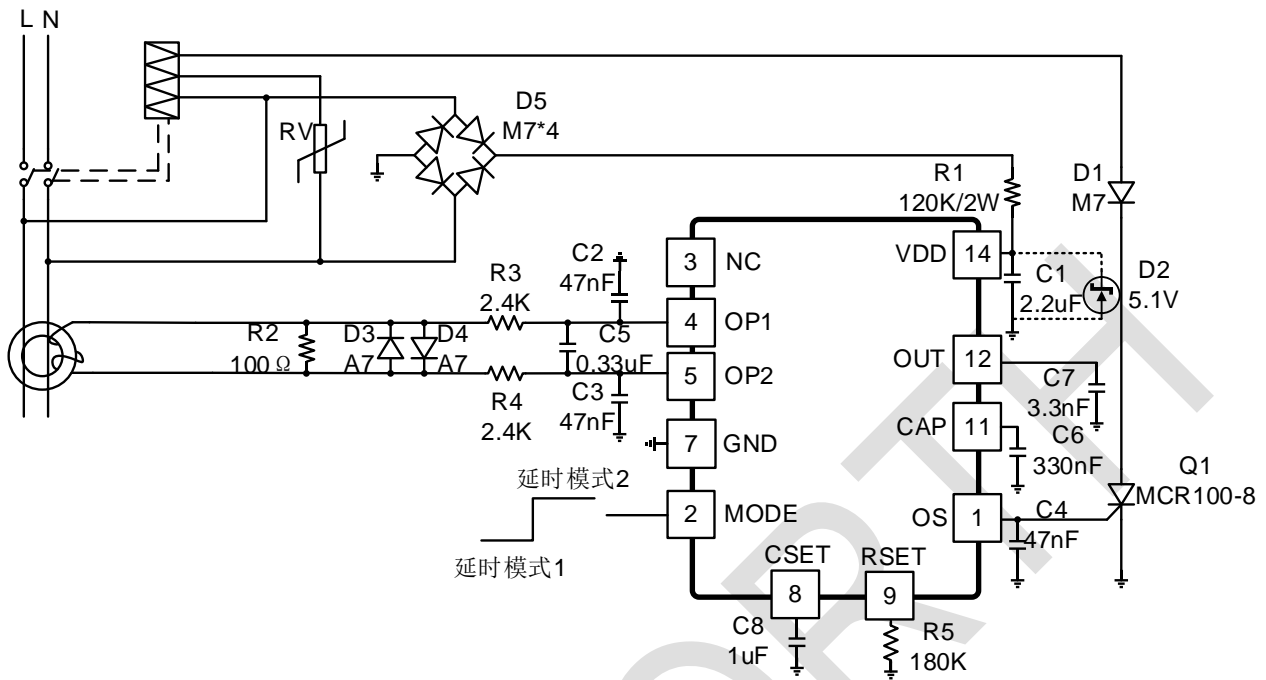
图 6.1 CN54124A 典型应用图
