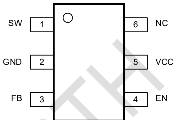
SOT-23-6L
